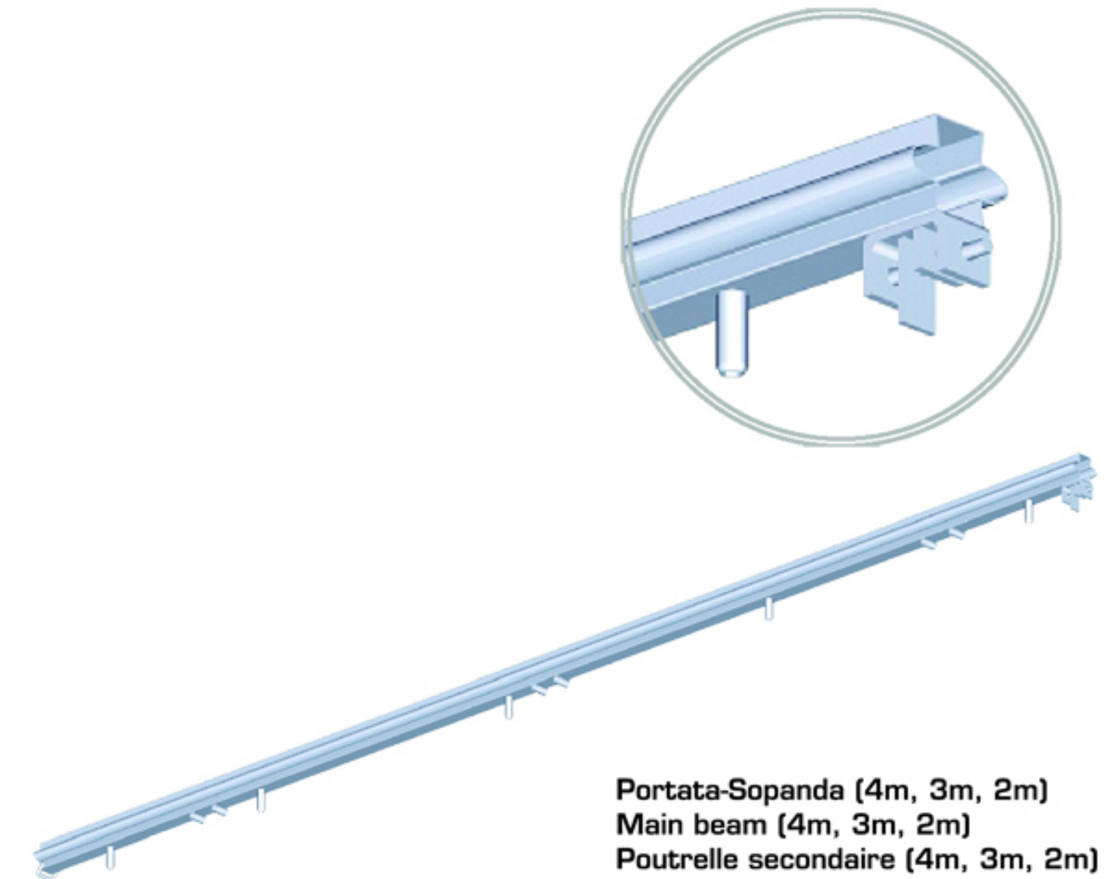
Montaje de guías y portata-sopandas. Mounting of transverse beams and main beams. Montage des poutrelles primaires et secondaires. Aufbau der Quer- und Längsträger. Montaggio di guide e portata-sopandas.
