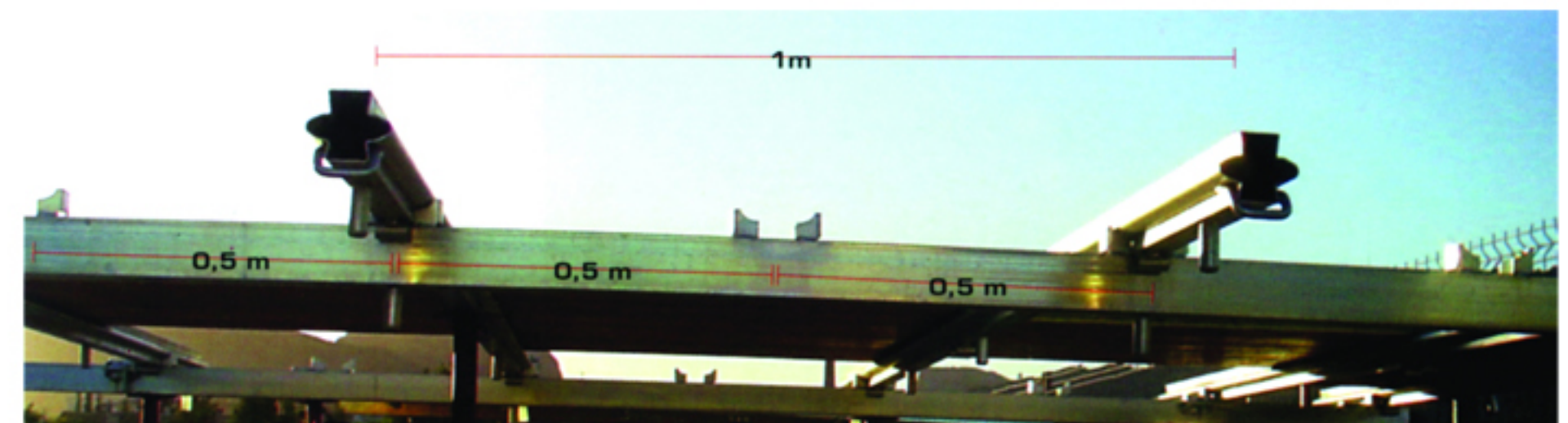
Montaje de guías y portata-sopandas. Mounting of transverse beams and main beams. Montage des poutrelles primaires et secondaires. Aufbau der Quer- und Längsträger. Montaggio di guide e portata-sopandas.
